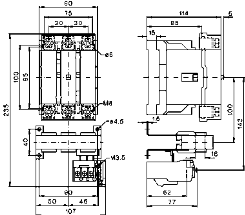
J7KN-200 + J7TKN-210
