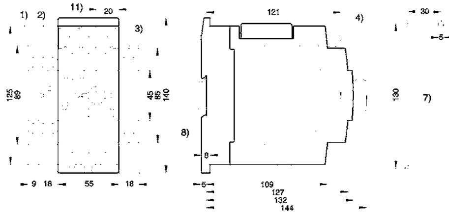
Circuit-breaker J7MN-100
