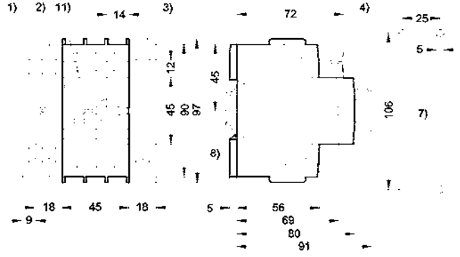
Circuit-breaker J7MN-25
