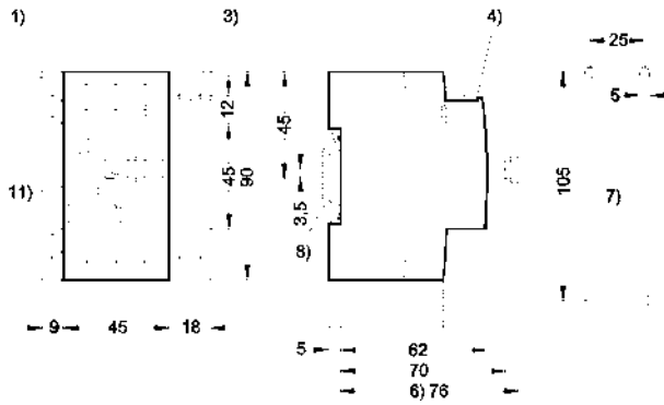
Circuit-breaker J7MN-50
