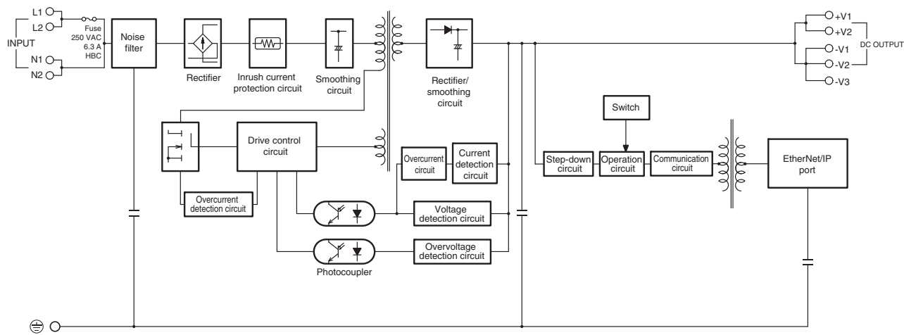
S8VK-X09024-EIP
